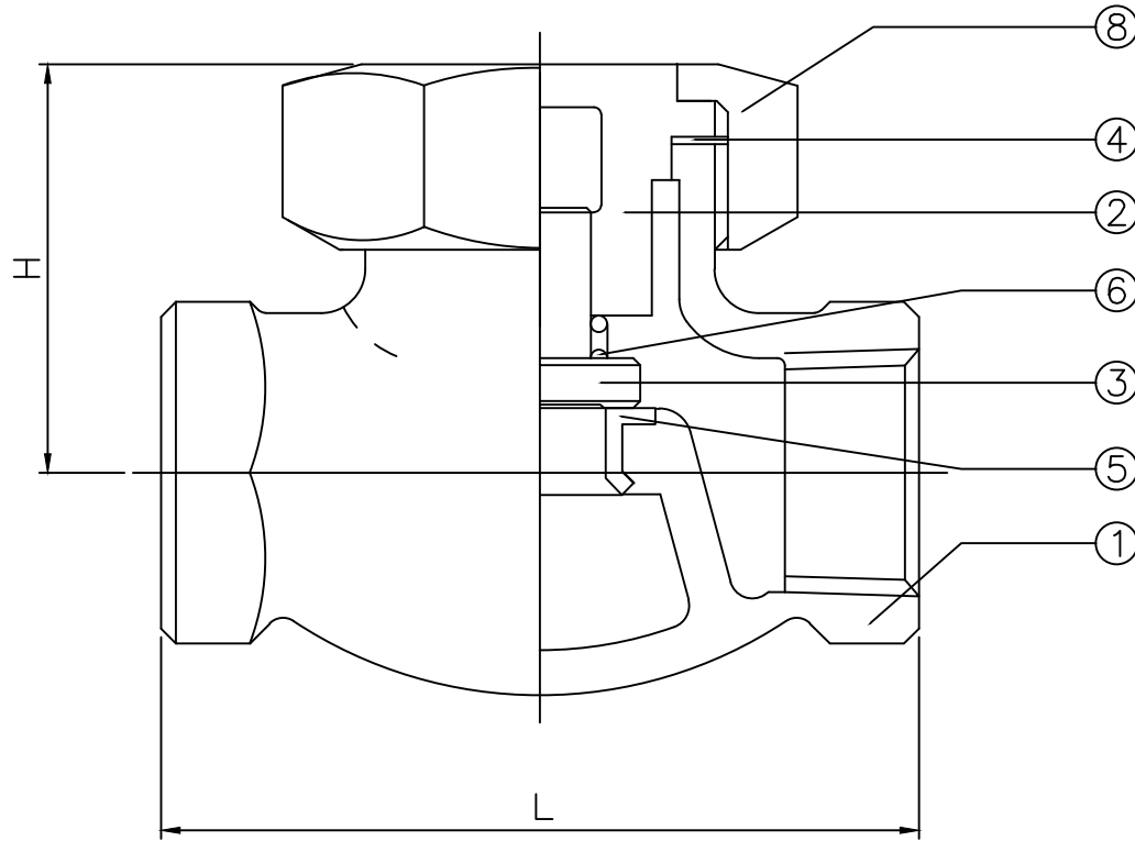
詳細尺寸 Dimension 單位 Unit: 公釐 mm
