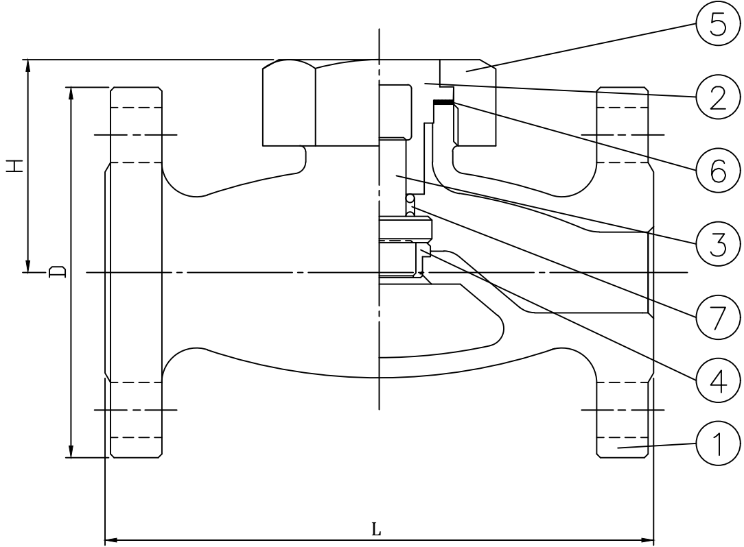
詳細尺寸 Dimension
